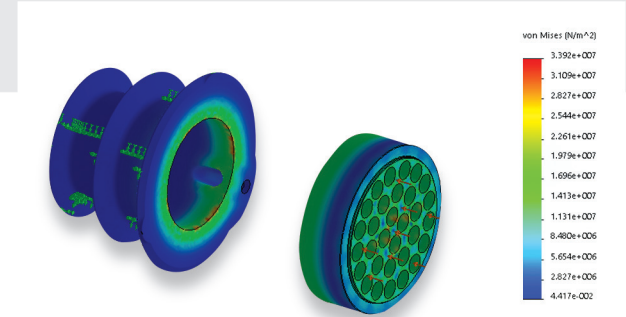
Germe Yük Test Simülasyonu Stressing Load Test Simulation
